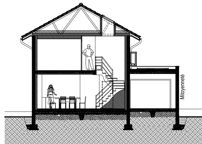
COUPE TRANSVERSALE
