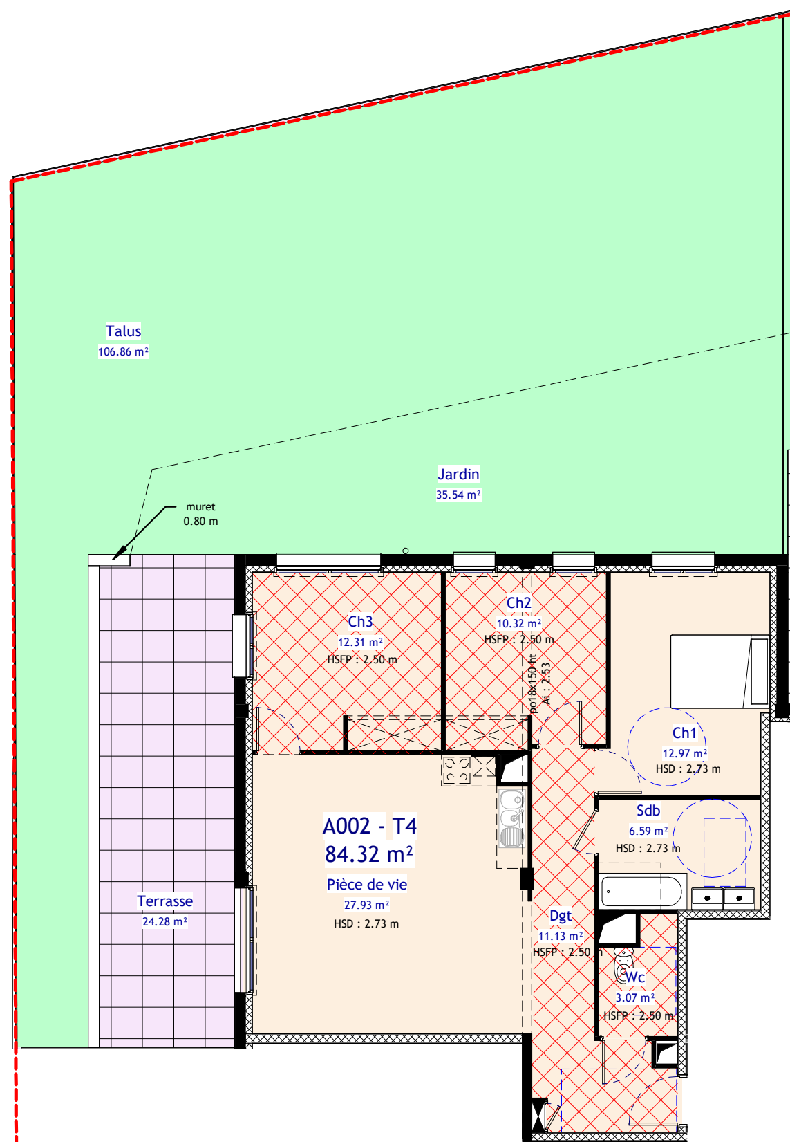
1 PDV A002 - GENERAL Ech : 1 : 100
