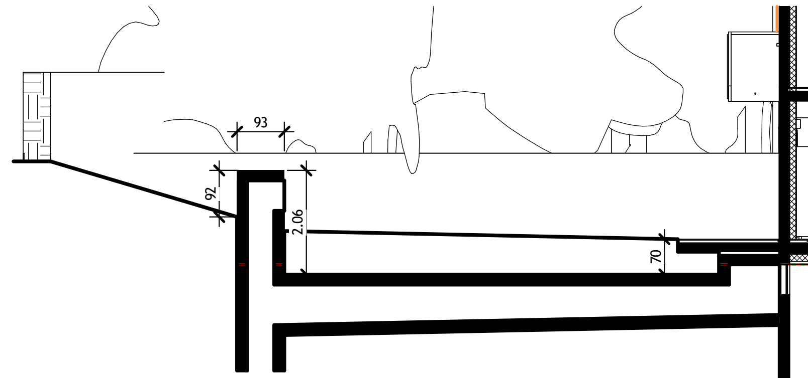
1 COUPE JARDIN A006 Ech : 1 : 75
