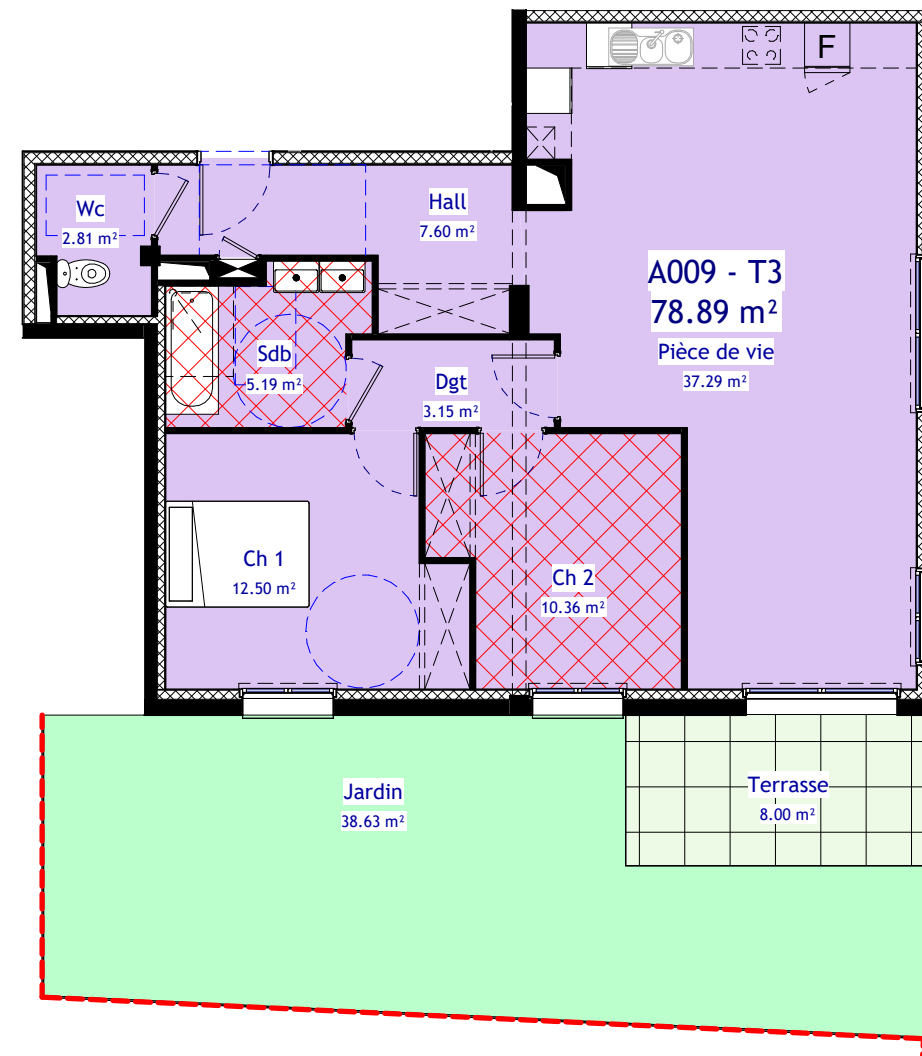
1 PDV A009 - GENERAL Ech : 1 : 100
